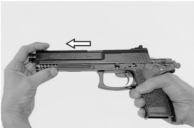
Verschluss abziehen Remove the slide
